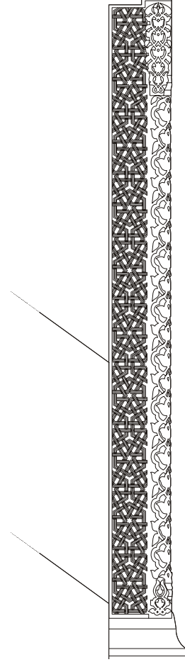
Şek.2- Balıkesir Zağanos Paşa Camisi Minberi. Söve ve köşe sütuncesi. (Çizim Aygül Uçar)
